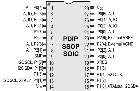
図 4. CY8C29466 28 ピン PSoC デバイス
