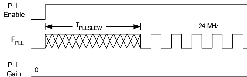
図 13. PLL ロック タイミング図
