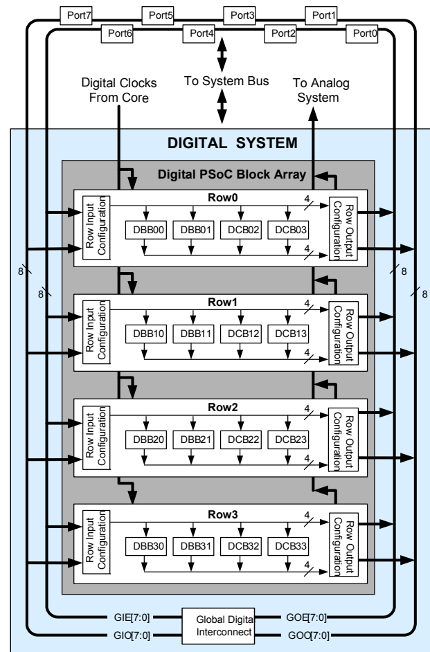
図 2. デジタル システムのブロック図
