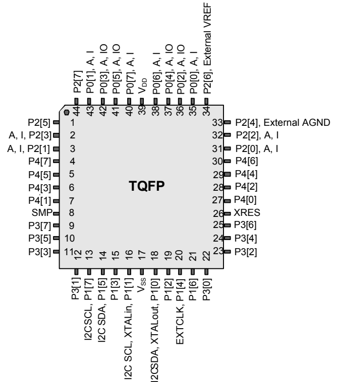
図 5. CY8C29566 44 ピン PSoC デバイス
