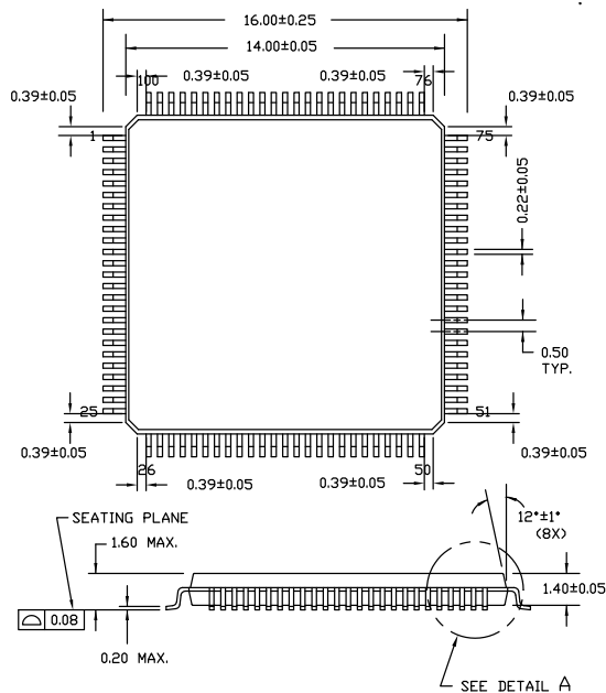
図 26. 100 ピン TQFP (14×14×1.4mm) パッケージ図、51-85048
