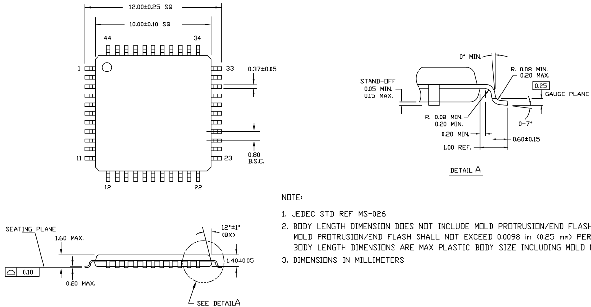
図 23. 44ピン TQFP (10×10×1.4mm) パッケージ図、51-85064
